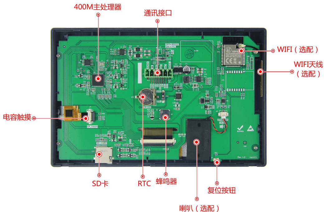
图 1-2 硬件配置图
