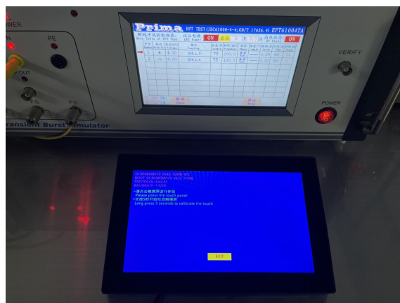
图 5-4 群脉冲测试图
